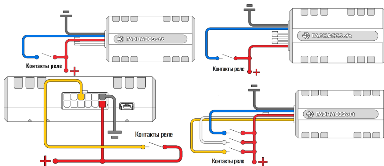
Рисунок 2.17 Варианты подключения дискретных датчиков
