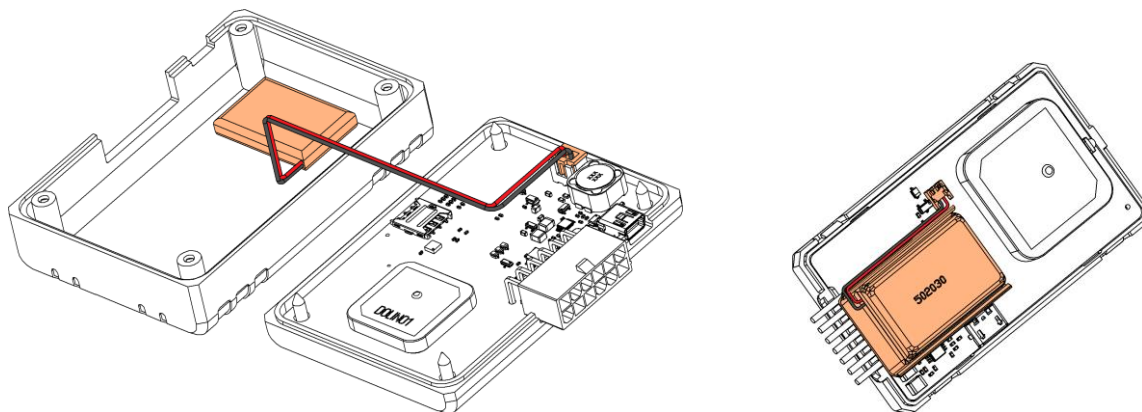
Рисунок 2.11 Установка аккумулятора (УМКа312 –слева; УМКа315 - справа)
