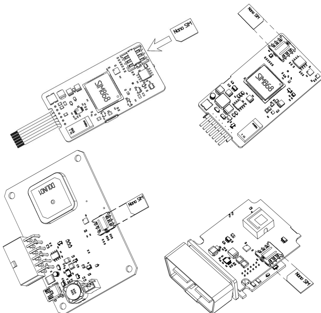
Рисунок 2.10 Установка SIM-карты
