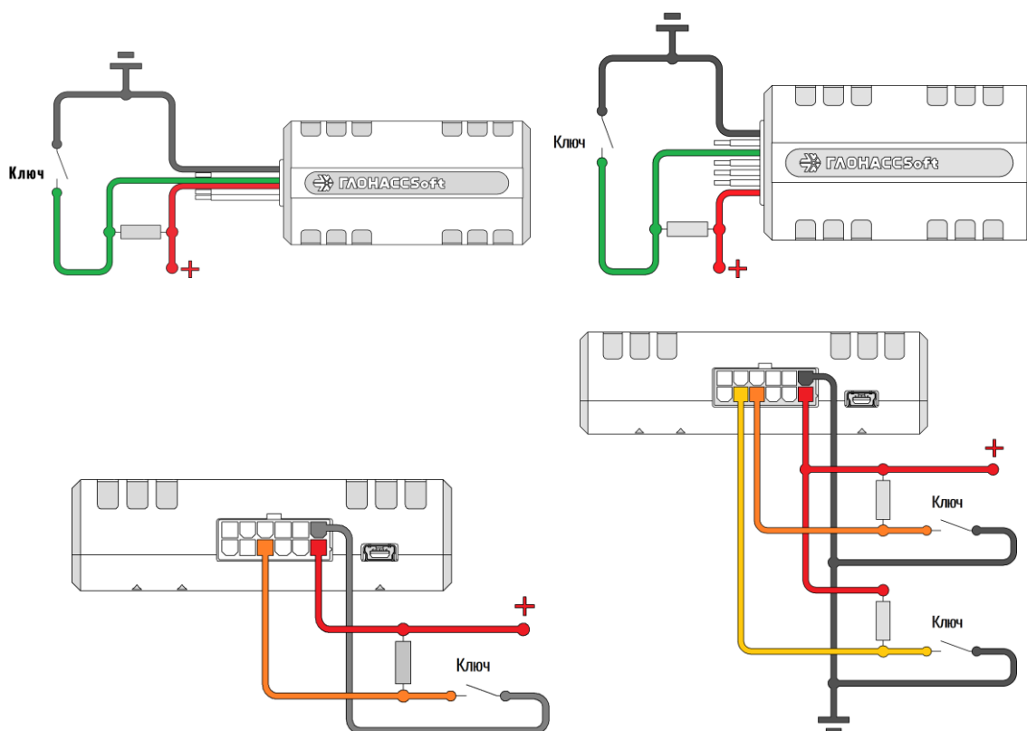
Рисунок 2.14 Подключение с подтяжкой к «+»
