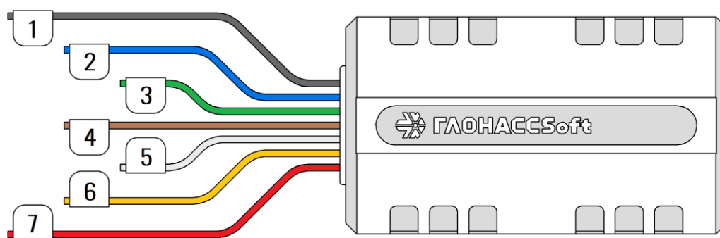
Рисунок 2.8 Нумерация выводов УМКа315
