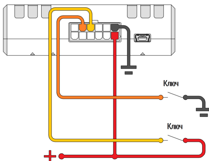
Рисунок 2.18 Варианты подключения дискретных датчиков к УМКа312v2
