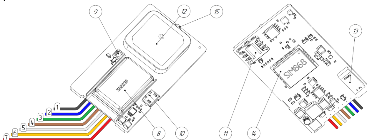
Рисунок 2.4 Основные элементы терминала УМКа315
