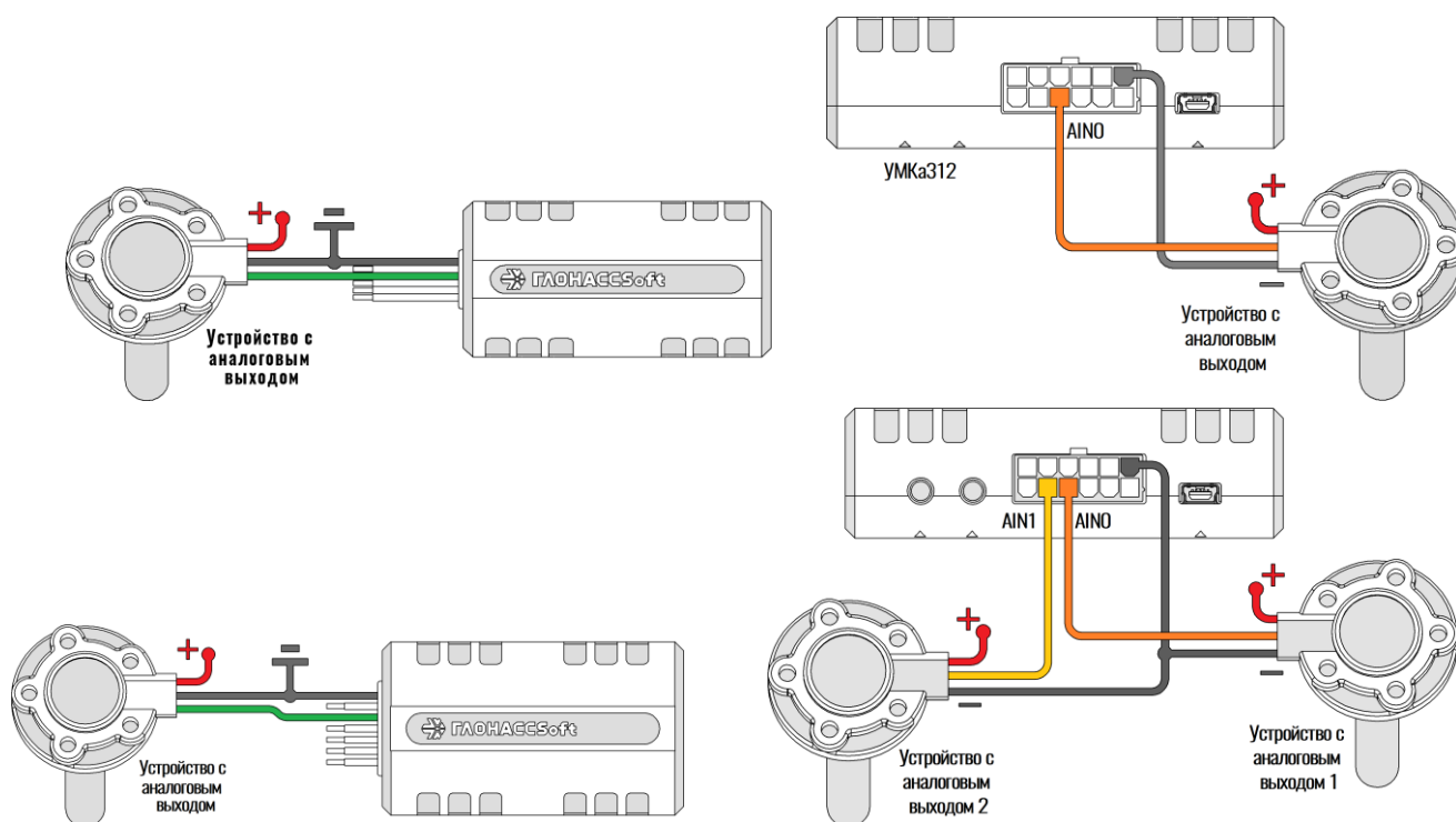
Рисунок 2.13 Подключение аналоговых источников УМКа310x – слева; УМКа312 – справа; УМКа315-снизу слева; УМКа 312v2 – снизу справа
