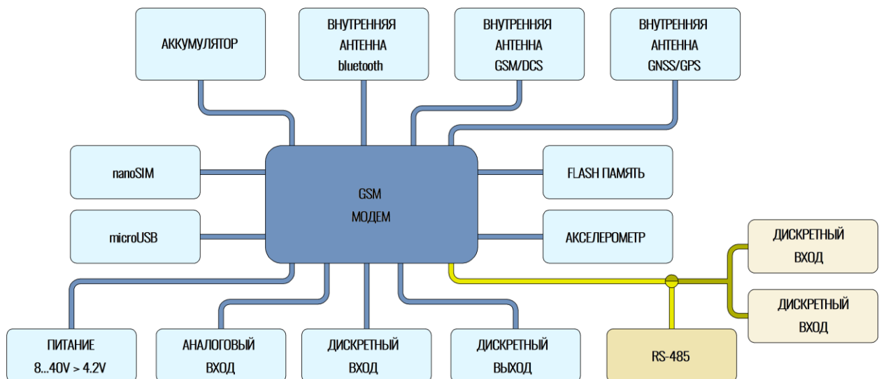
Рисунок 1.5 Блок-схема навигационного терминала УМКа315
