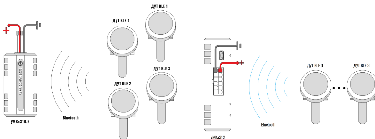
Рисунок 2.23 Подключение ДУТ по BLE
