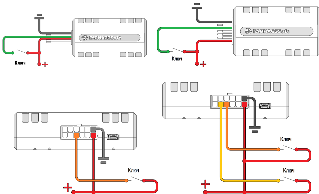
Рисунок 2.15 Подключение с подтяжкой к «-»
