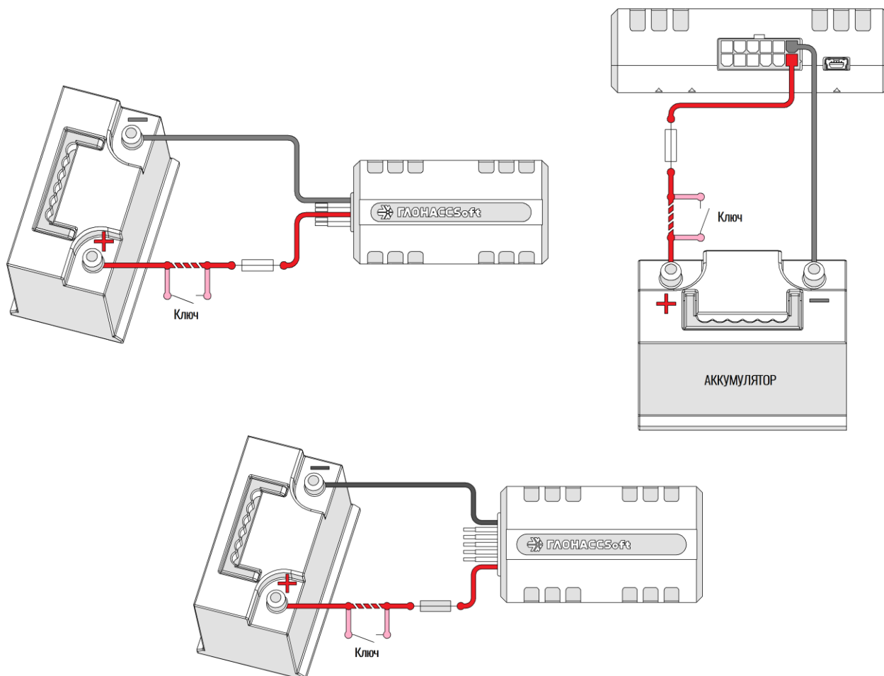
Рисунок 2.12 Подключение питаниям
