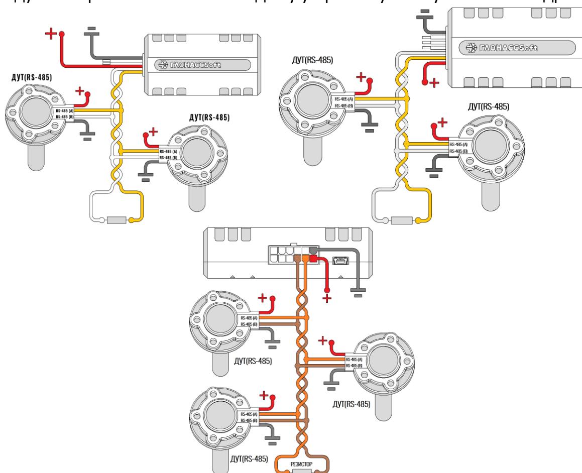
Рисунок 2.21 Подключение ДУТ по интерфейсу RS-485
