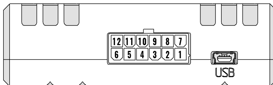
Рисунок 2.7 Нумерация выводов УМКа312х
