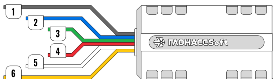
Рисунок 2.5 Нумерация выводов УМКа310х
