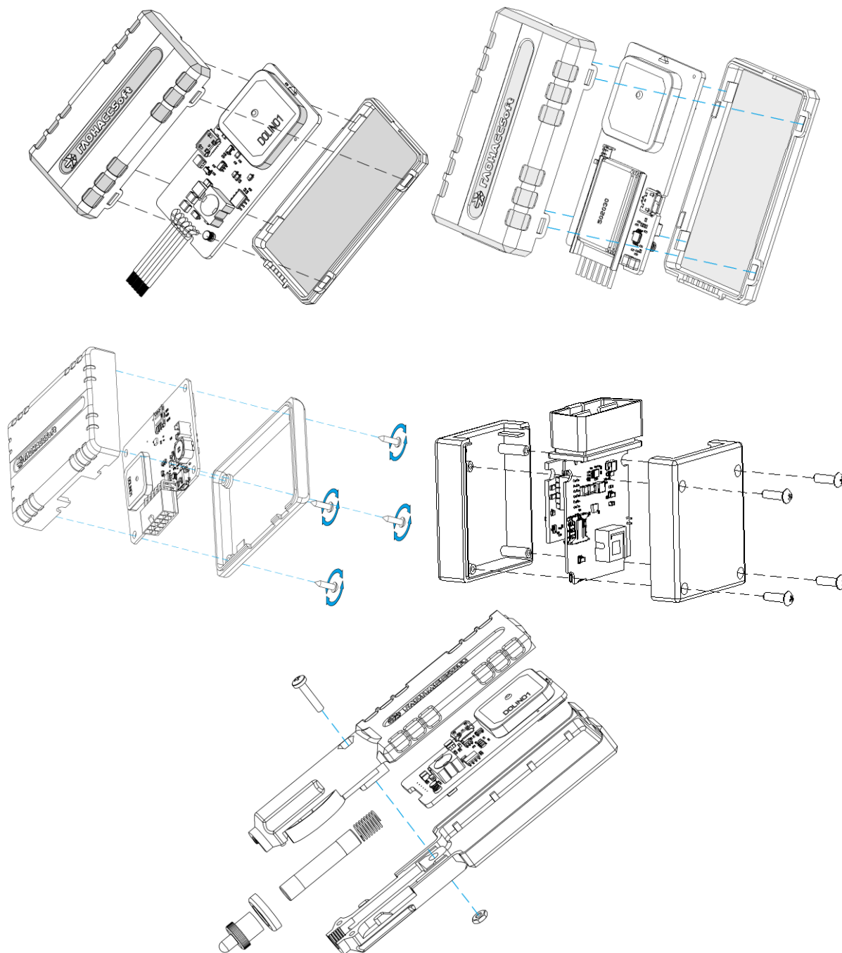
Рисунок 2.9 Вскрытие корпуса терминала
