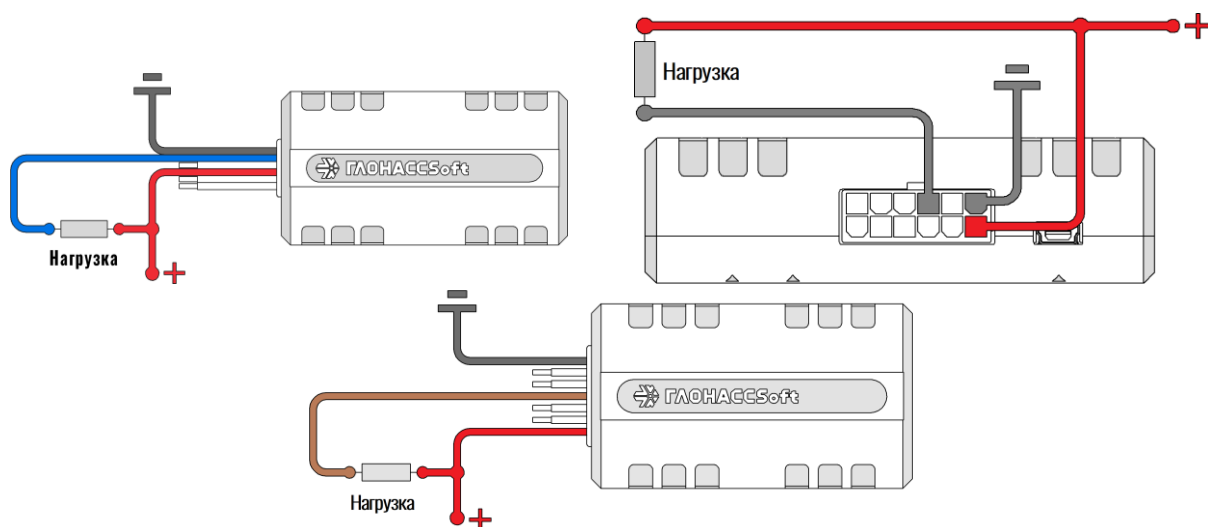
Рисунок 2.19 Подключение маломощной нагрузки
